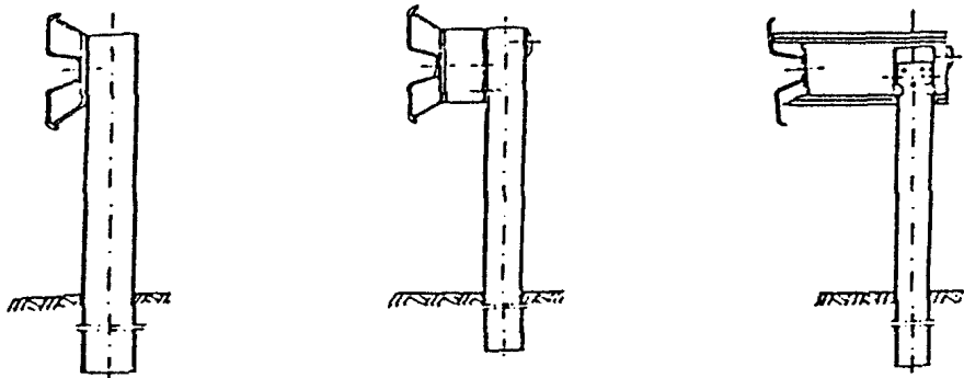
c) wysięgnikowa
